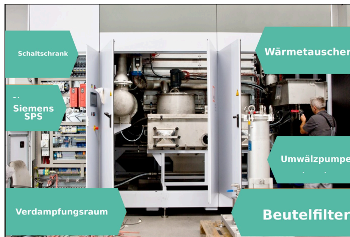
MVR-Verdampfermodul (Beispielfoto)
